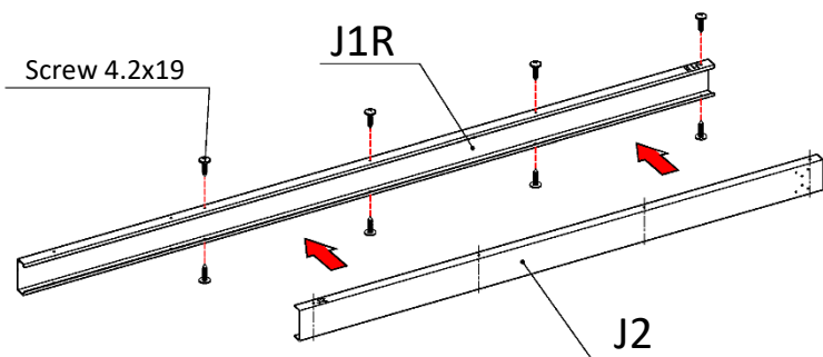
Longitudinal beam J1R+J2
