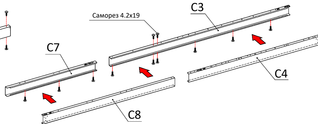
Торцевая балка C3+C4+C7+C8
