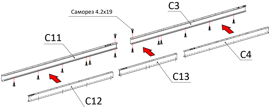
Торцевая балка C3+C4+C11+C12+C14
