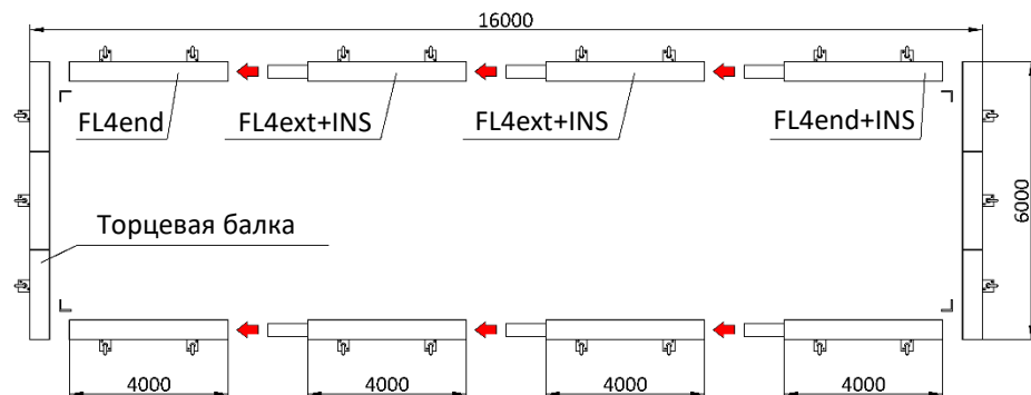
Опорная рама 6000x16000
