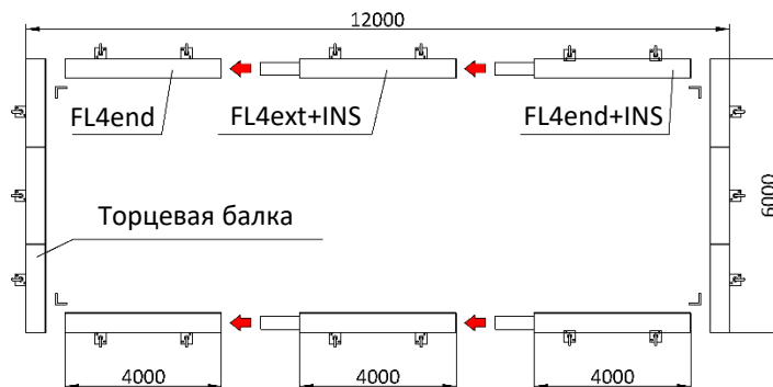
Опорная рама 6000x12000
