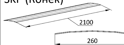
СКР (Конек)
