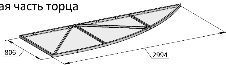
Вставка торца правая
