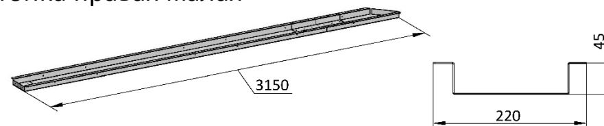
Стойка правая малая
