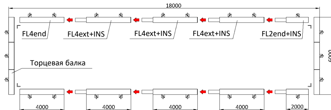
Опорная рама 6000x18000
