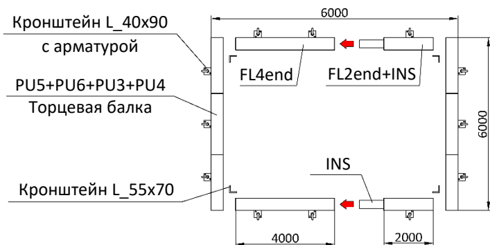
Опорная рама 6000x6000
