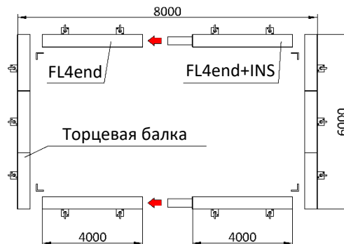
Опорная рама 6000x8000
