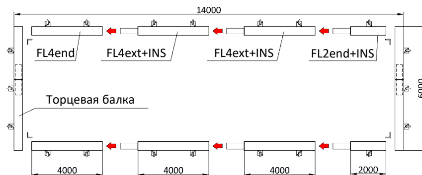
Опорная рама 6000x14000
