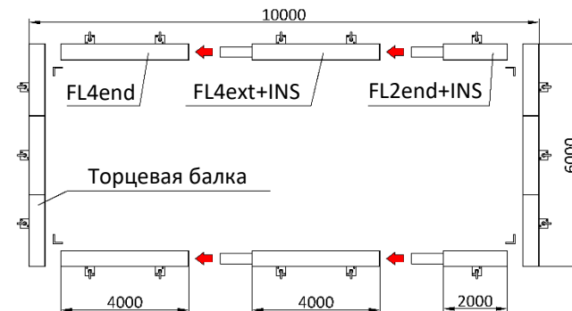
Опорная рама 6000x10000
