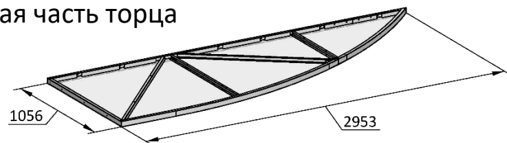
Вставка торца правая
