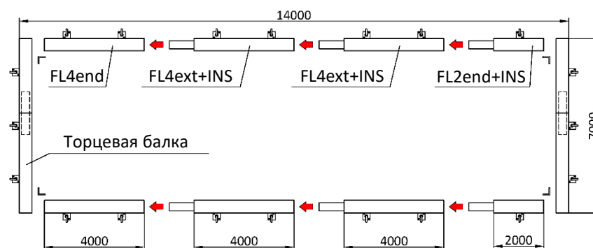
Опорная рама 7000x14000
