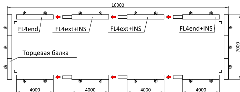
Опорная рама 7000x16000
