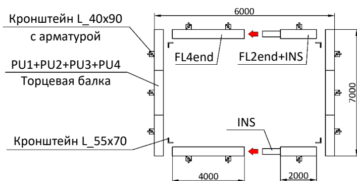
Опорная рама 7000x6000
