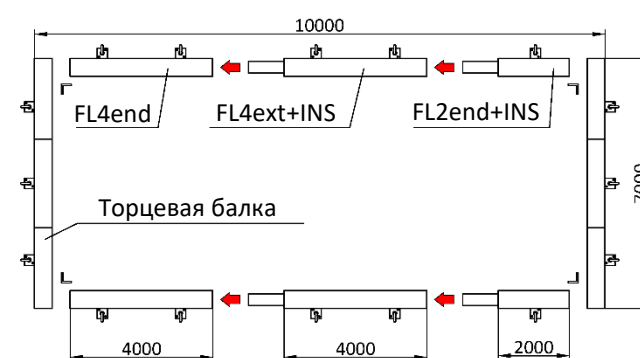
Опорная рама 7000x10000
