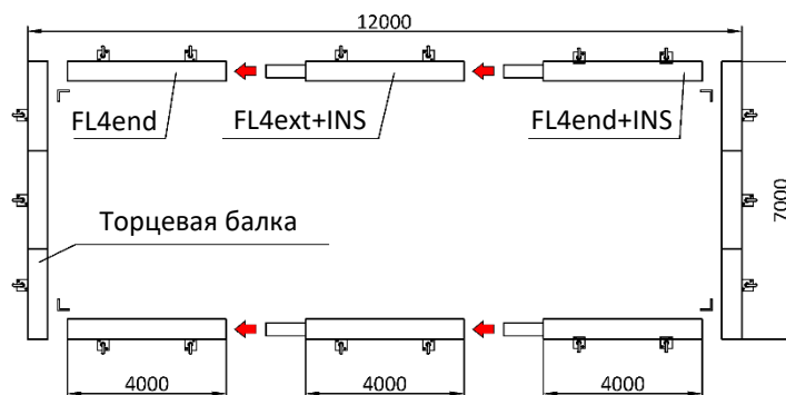
Опорная рама 7000x12000
