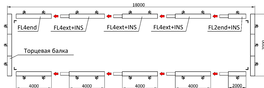
Опорная рама 7000x18000
