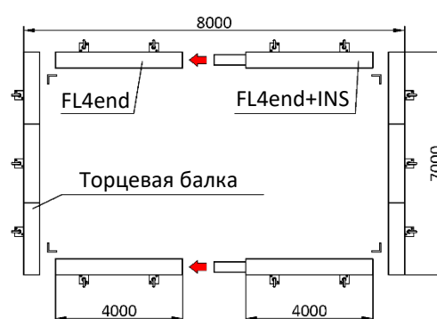
Опорная рама 7000x8000
