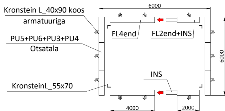
Toestusraam 6000x6000
