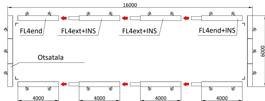
Toestusraam 6000x16000
