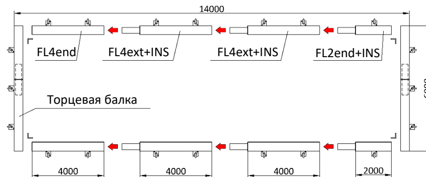
Toestusraam 6000x14000
