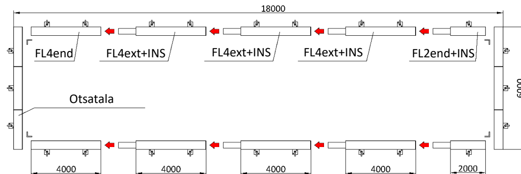
Toestusraam 6000x18000
