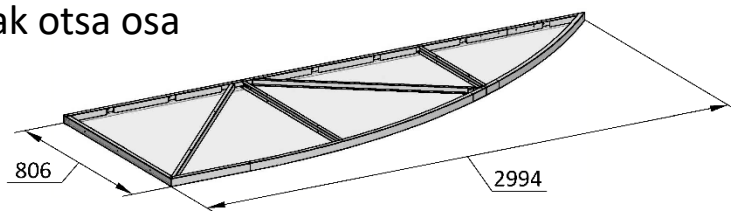
Parem otsa sisetük
