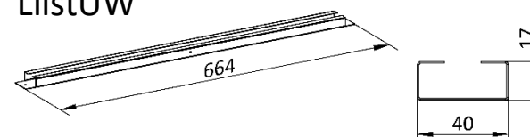
SKP (Hari)
