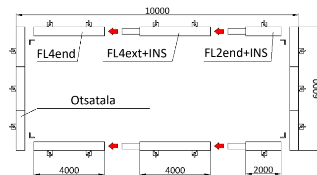
Toestusraam 6000x10000
