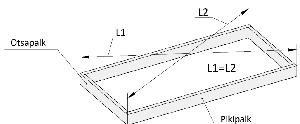
E Toestusraami paigaldamise nõuded
