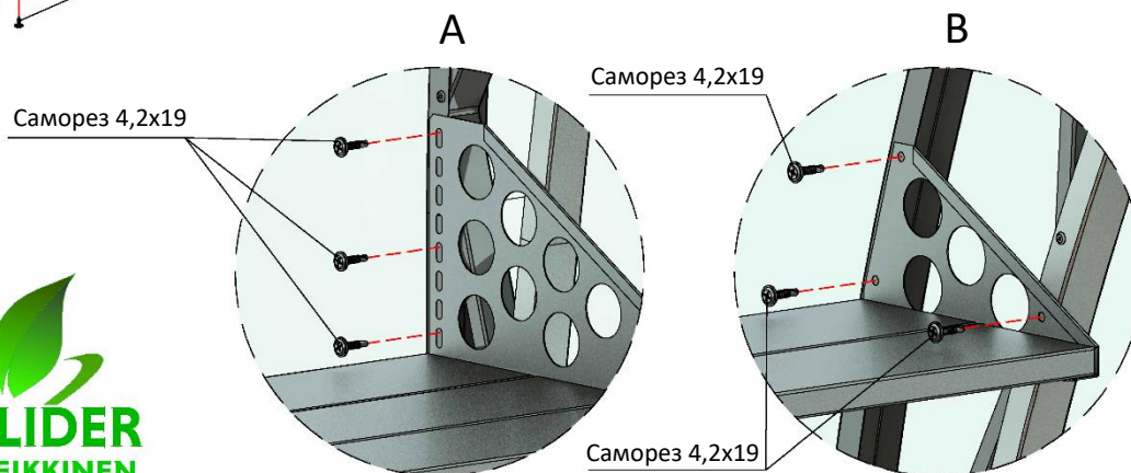
Установка полок
