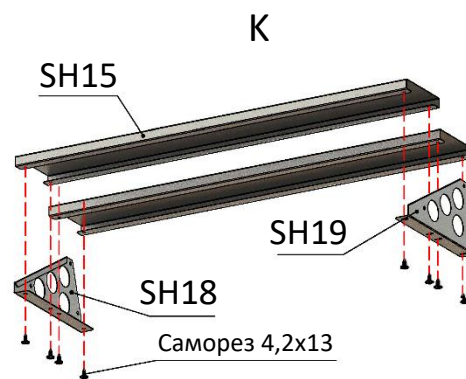
Установка полок
