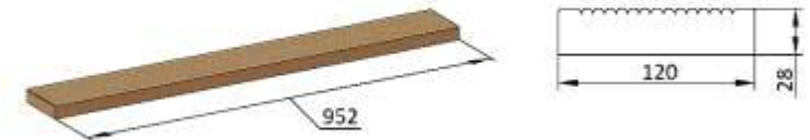
Kinnitusedetailid
